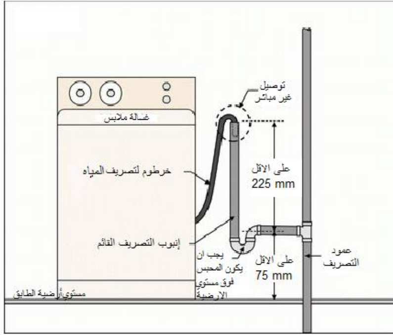
الشكل 7-3/ أنبوب التصريف القائم لغسالة الملابس الالية
