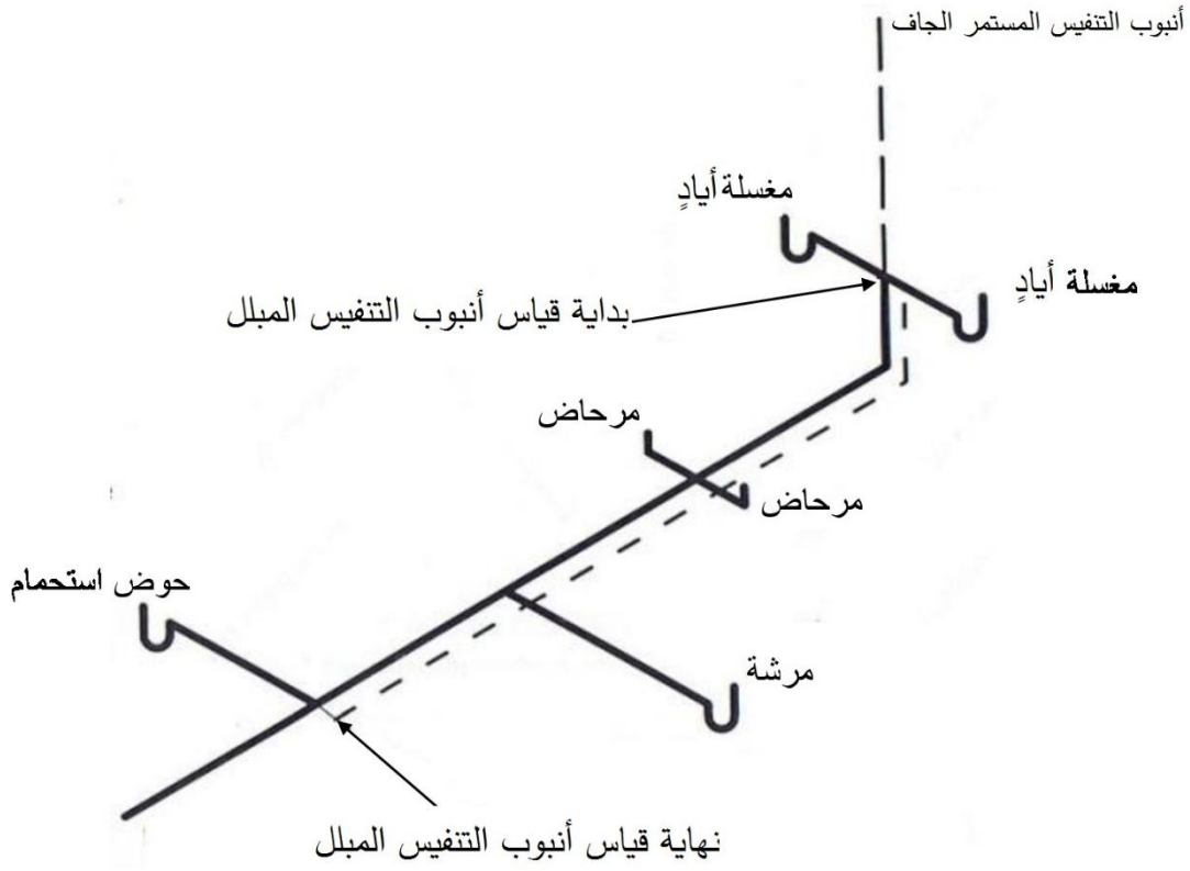
الشكل 12-9/1: أنبوب التنفيس المبلل الأفقي
