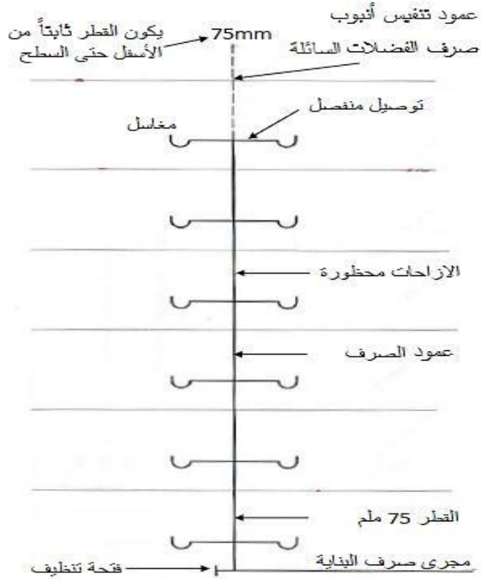
الشكل 12-10: عمود تنفيس أنبوب صرف الفضلات السائلة
