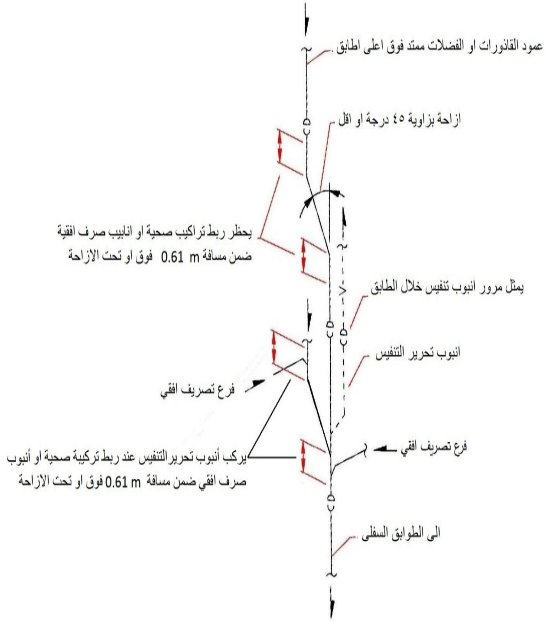
الشكل 10-1: ربط فرع المجاري الافقي ضمن مسافة 0.61 م فوق أو تحت الازاحة العمودية
