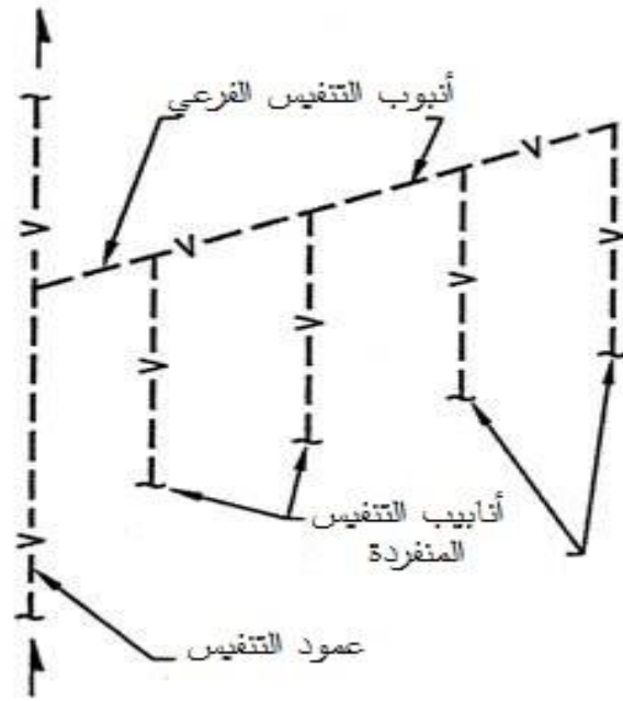
الشكل 1-2/2: أنبوب التنفيس الفرعي
