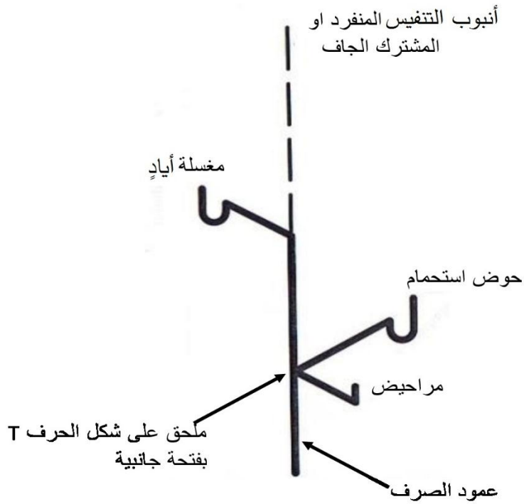
الشكل 12-9/2: أنبوب التنفيس المبلل العمودي
