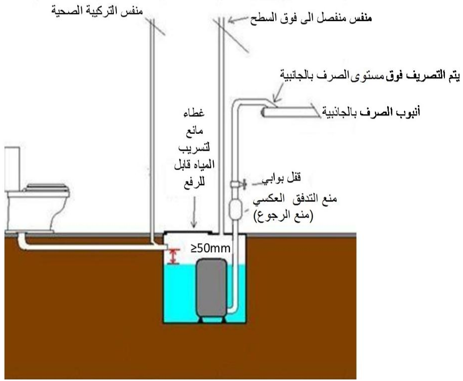
الشكل 11-2/4: تركيب قاذفة مياه الصرف الصحي
