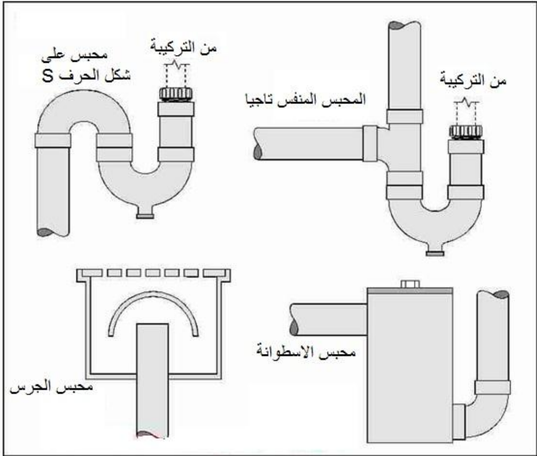
الشكل 7-5: المحابس المحظورة
