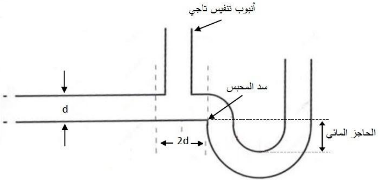
الشكل 12-6: التنفيس التاجي
