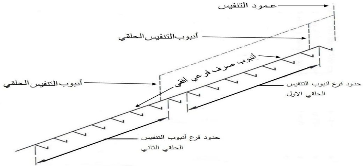
الشكل 12-11/2: تفاصيل ربط أنابيب تنفيس حلقيّة متعددة على التوالي
