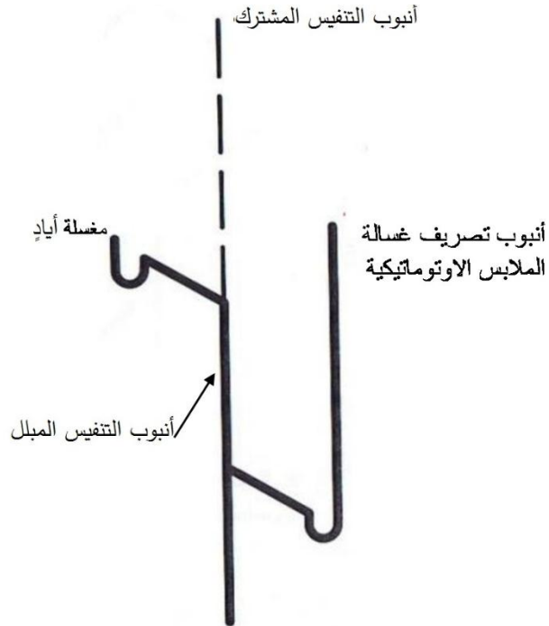
الشكل 12-2/8: أنبوب التنفيس المشترك
