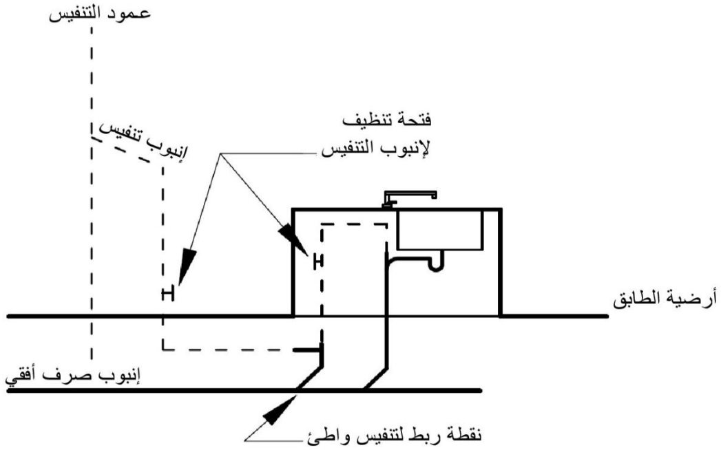
الشكل 12-1/12: تفاصيل أنبوب الصرف والتهوية المشترك
