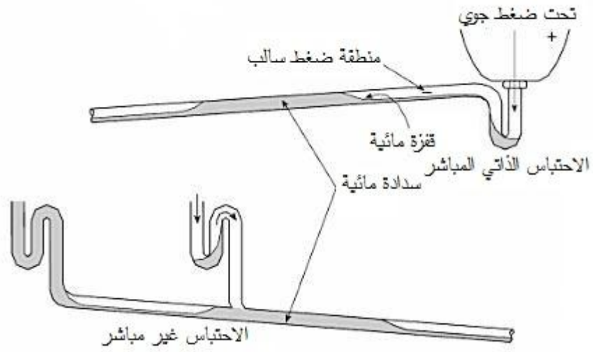
الشكل 7-5/2: الاحتباس غير المباشر
