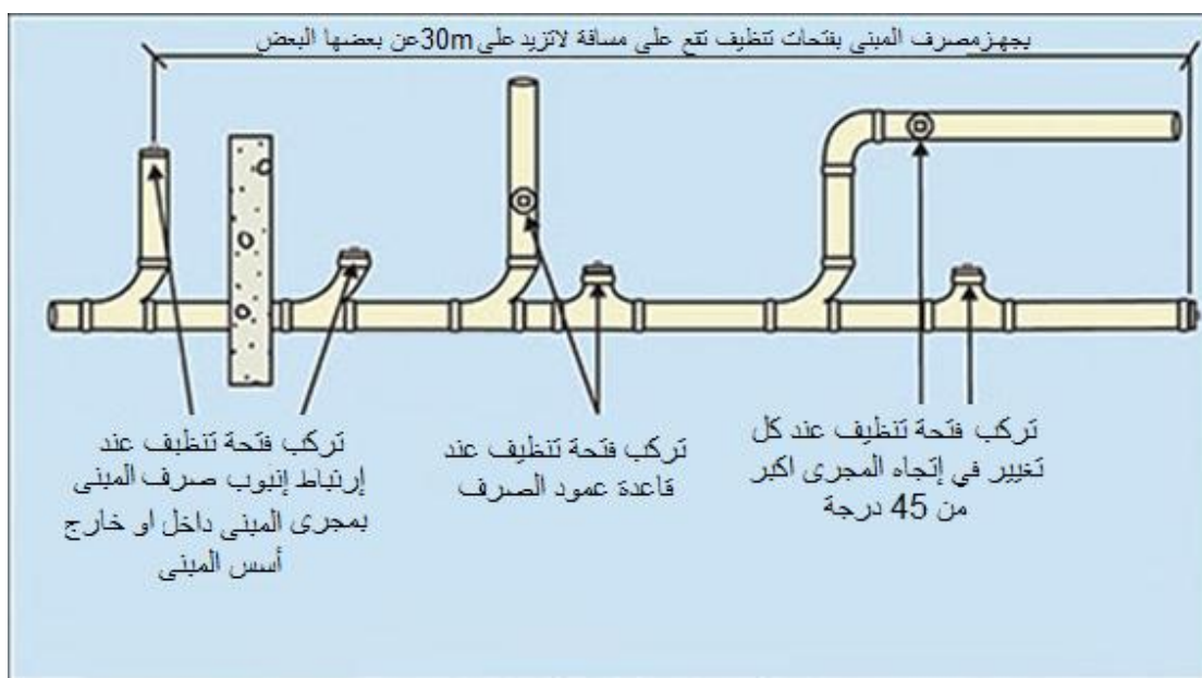
الشكل 8-1/2: بعض مواقع فتحات التنظيف
