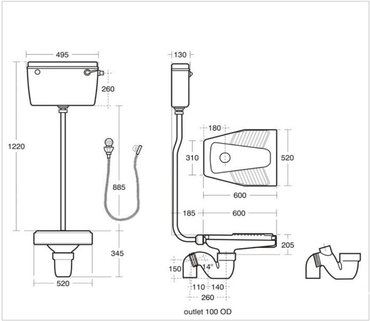
الشكل 6-1/5 : المراحيض الشرقية أو العربية (الابعاد بالمليمترات)
