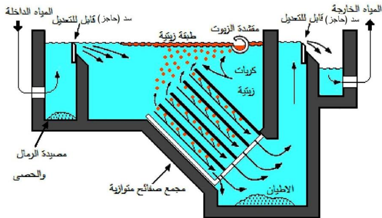
الشكل 13-1/2: جهاز عزل الزيوت والرمل والاطيان
