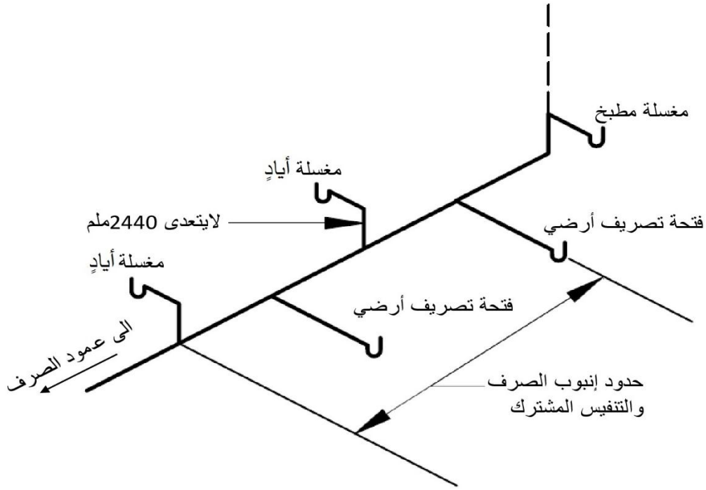
الشكل 12-1/12: تفاصيل أنبوب الصرف والتهوية المشترك
