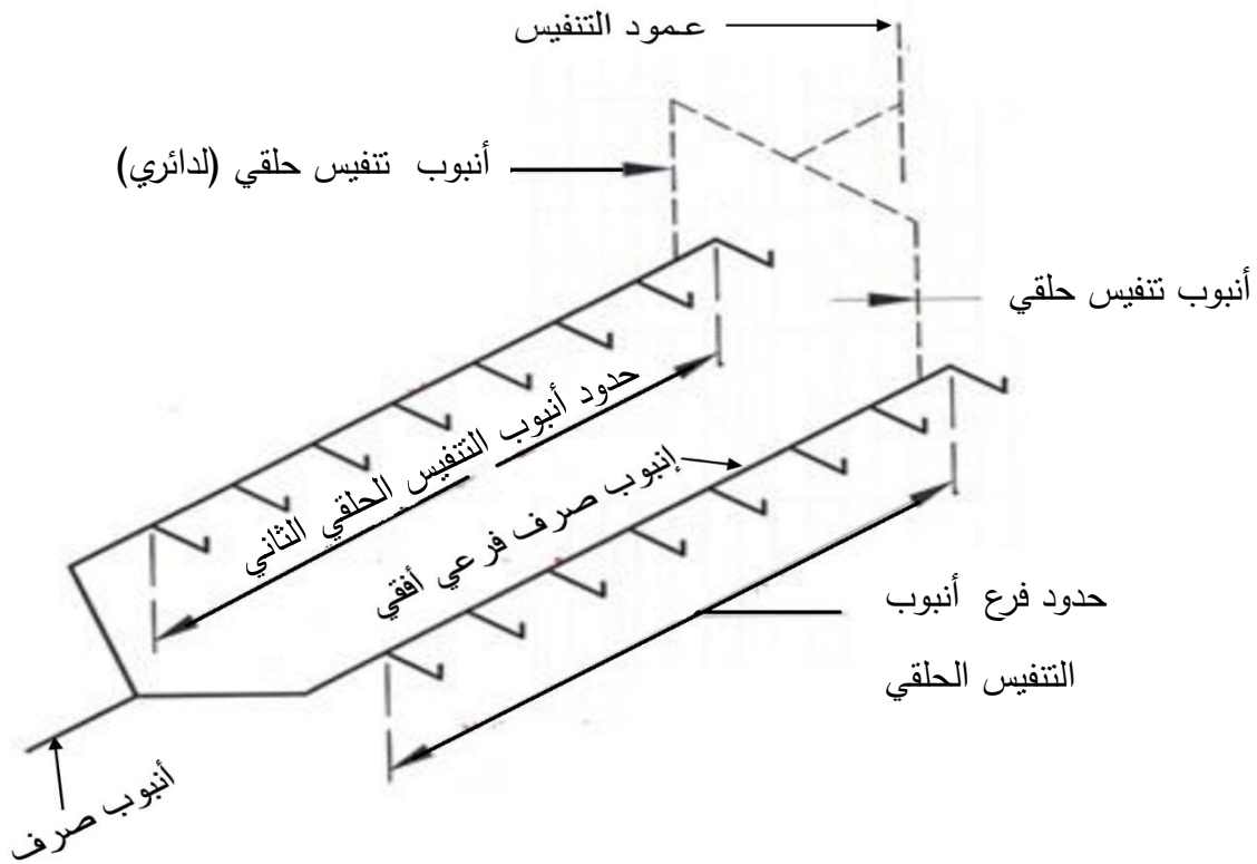
الشكل 12-11/3: تفاصيل ربط أنابيب تنفيس حلقيّة على التوازي
