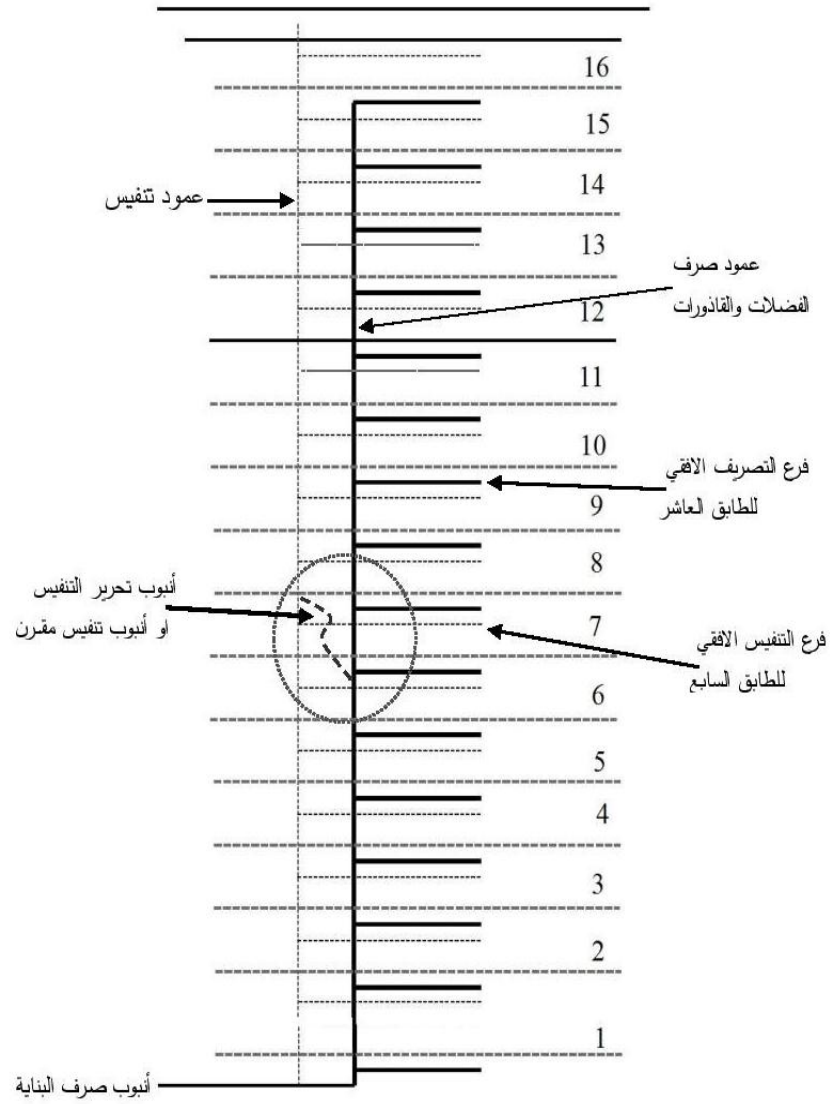
الشكل 12-14: تفاصيل ربط أنبوب تحرير التنفيس في الأبنية التي تزيد على عشرة طوابق
