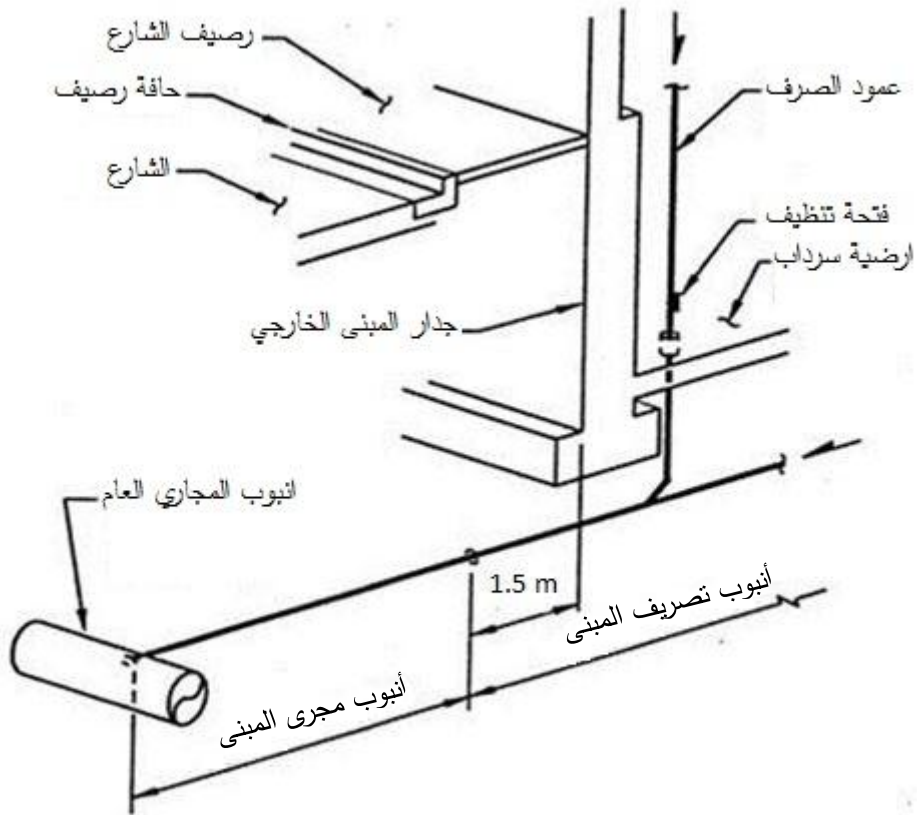
الشكل 1-3/2: أنبوب الصرف الصحي للمبنى
