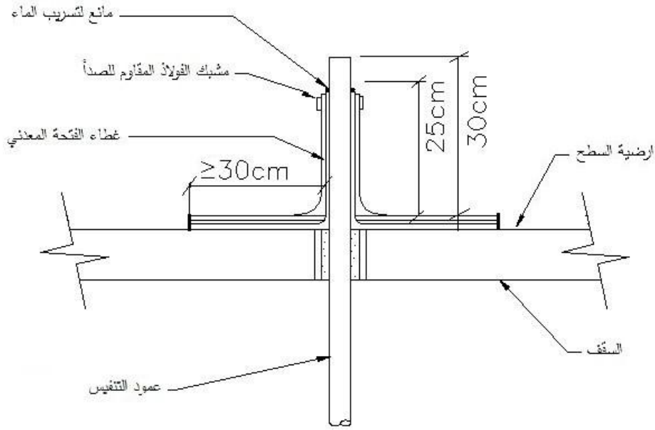
الشكل 2-10: تفاصيل تغليف نهايات عمود التهوية فوق سطوح الابنية
