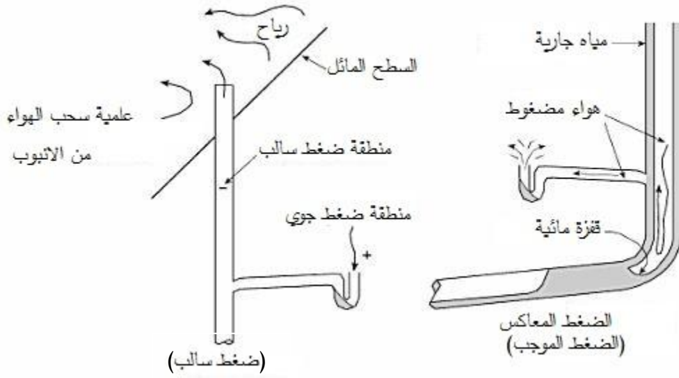
الشكل 7-6/1: الضغط المعاكس
