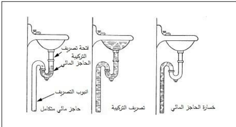
الشكل 7-1: الاحتباس الذاتي المباشر
