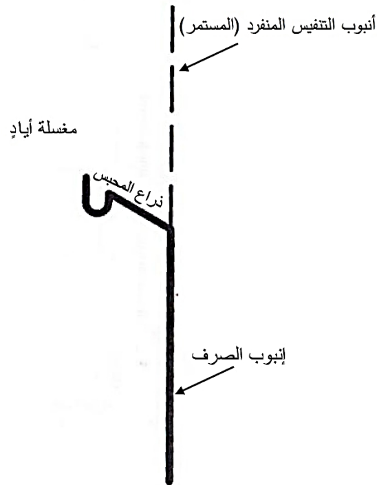
الشكل 12-7: التنفيس المنفرد (المستمر)
