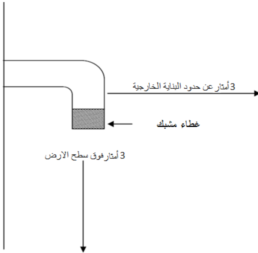
الشكل 12-4/1: موقع أنابيب التهوية بالسطح
