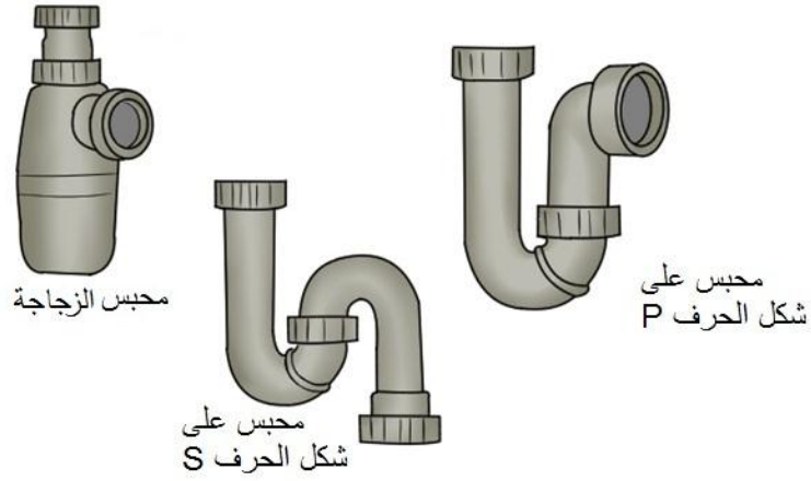
الشكل 7-4/ اشكال المحابس
