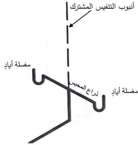
الشكل 12-1/8: التنفيس المشترك
