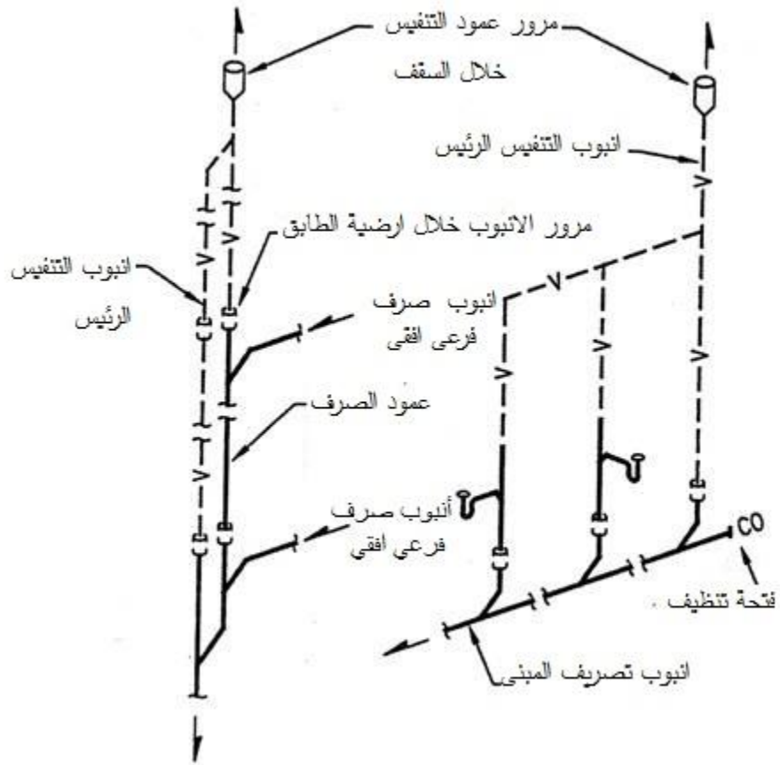
الشكل 1-2: أنبوب التهيف الرئيس
