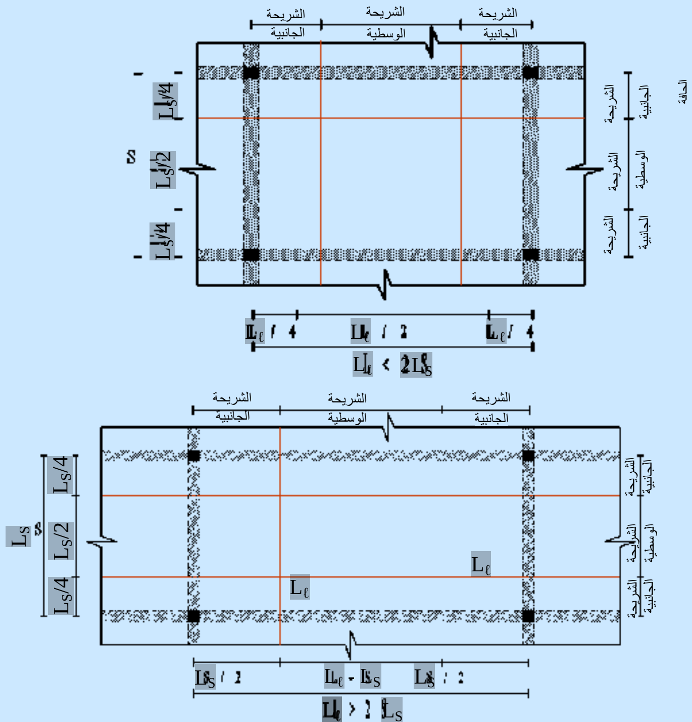
شكل (4-10) توزيع الشرائح الوسطية والجانبية الخاصة بالبلاطات المصممة بطريقة معاملات العزوم
