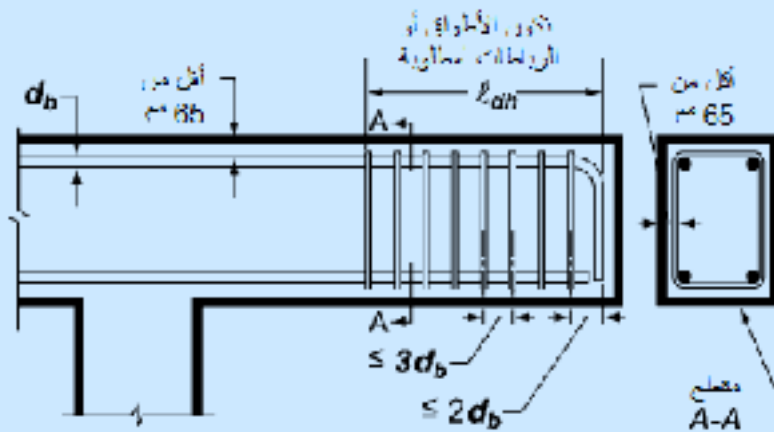
شكل (9-4) غطاء الحماية الخرساني المطلوب
