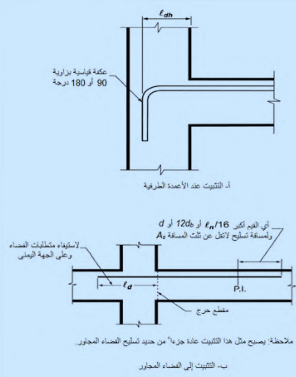
شكل (9-9) أطوال التثبيت لحديد تسليح العزوم السالبة
